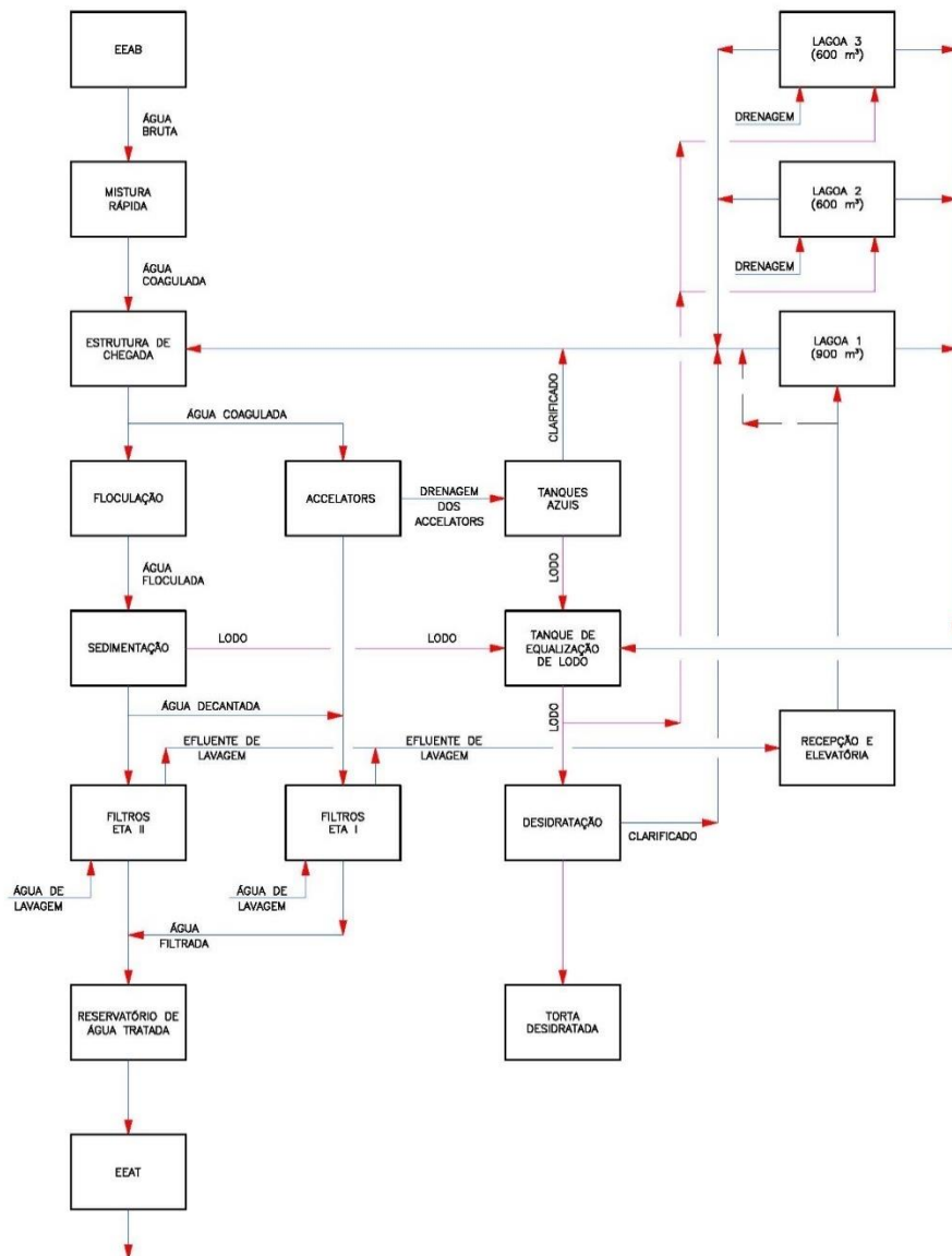
FIGURA 5.1 ETA JUTURNAIBA FLUXOGRAMA DAS CORRENTES LÍQUIDAS
