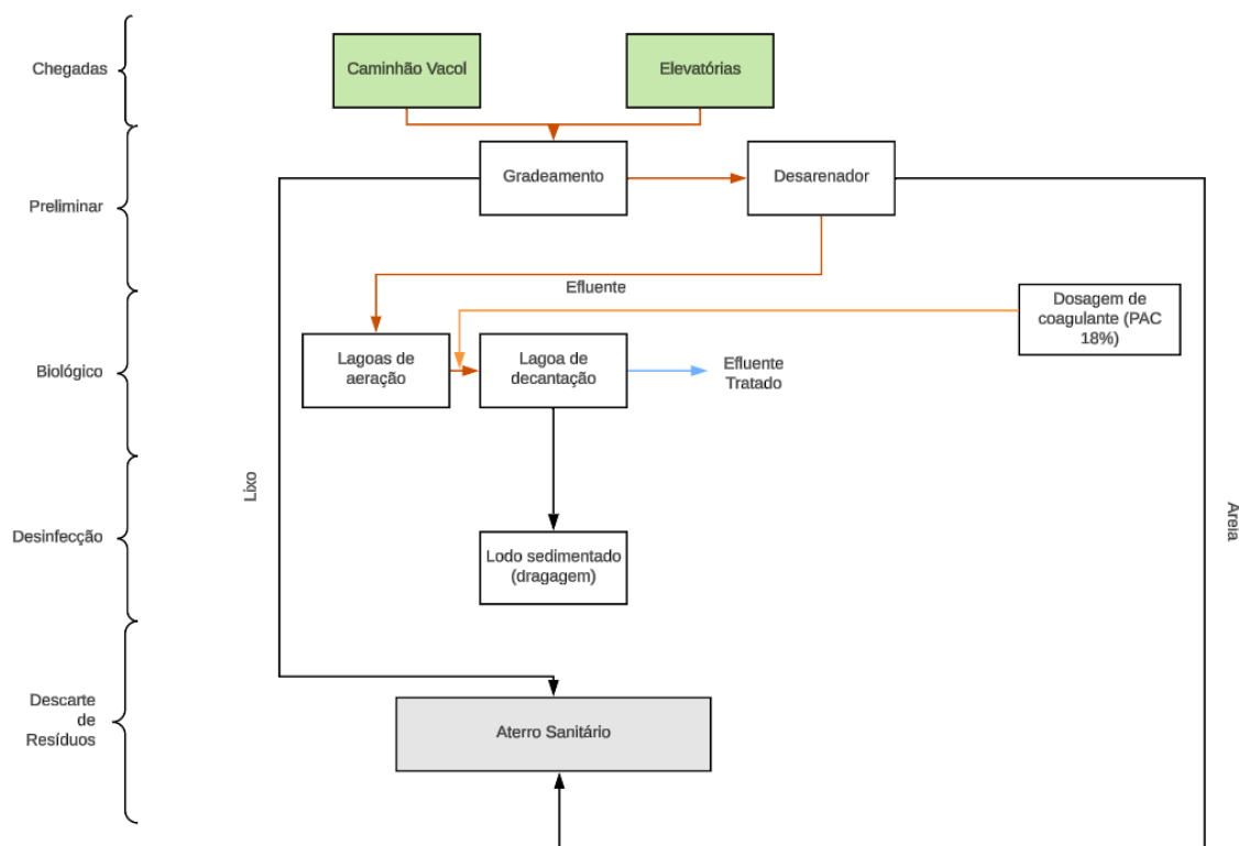
Figura 67 – Fluxograma ETE Jardim Esperança.
