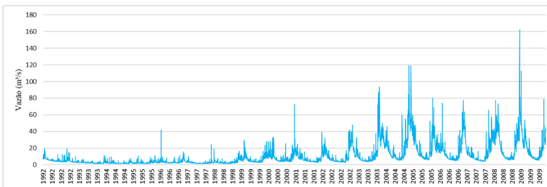
Figura 28 - Hidrograma de vazões simuladas para a sub-bacia da Lagoa de Araruama.
